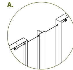
BEFESTIGUNG ZWISCHENPFOSTEN
