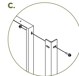
BEFESTIGUNG ENDEN ECKPFOSTEN
