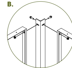
BEFESTIGUNG ECKPFOSTEN
